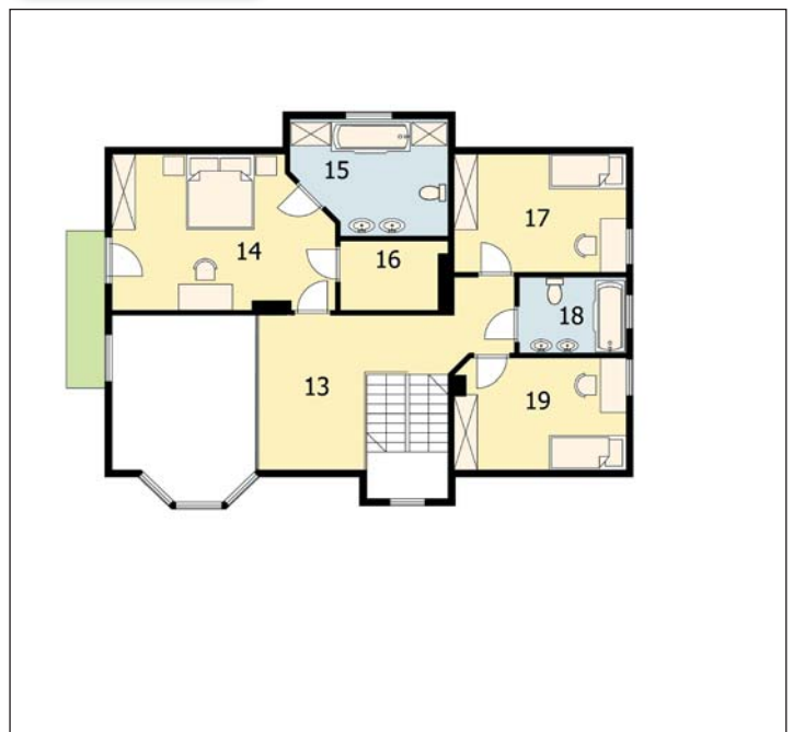
rzut poddasza
