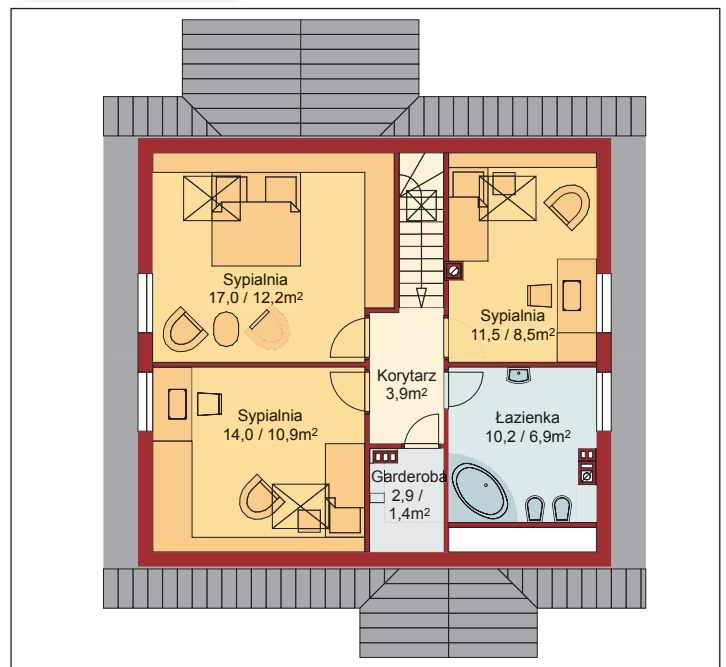
rzut poddasza
