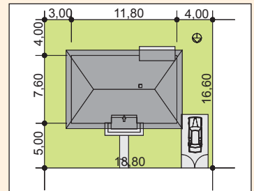
rzut na działce
